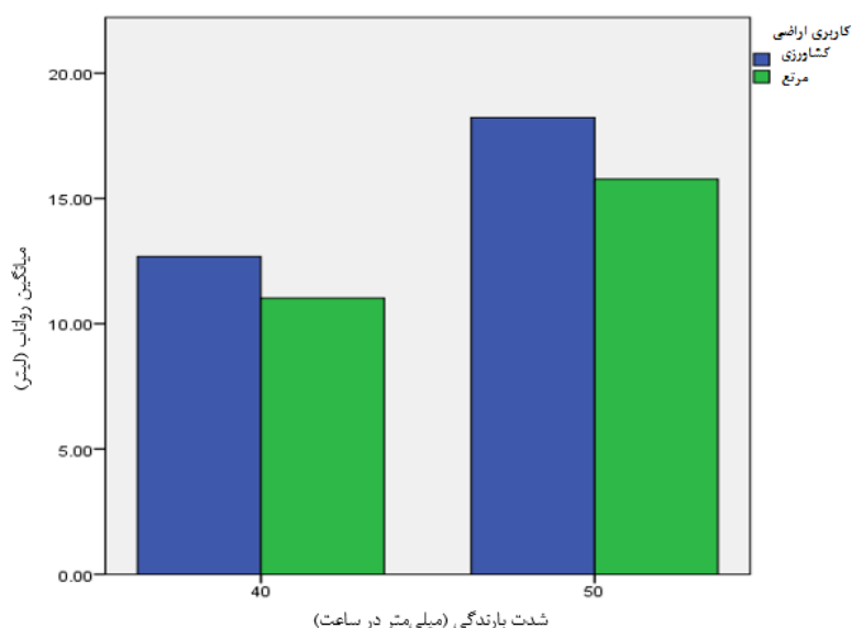
شکل ۴- زیرمجموعه‌های همگن داده‌های رواناب در شدت باران و کاربری‌های مختلف.
