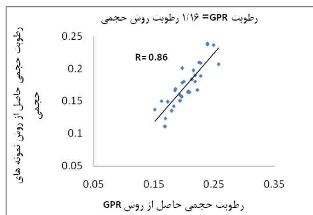
شکل ۷- رابطه‌ی بین رطوبت‌های حجمی محاسبه‌شده با روش GPR در مقایسه با روش نمونه‌های حجمی
